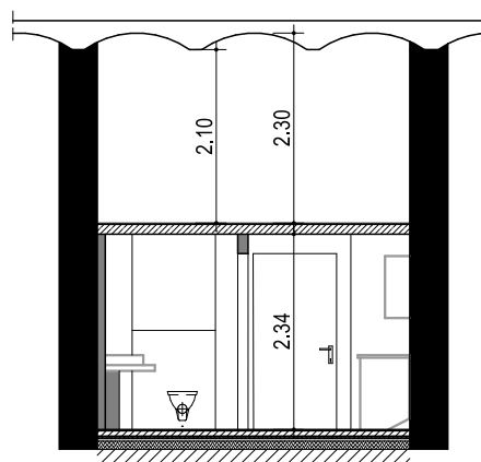
Prinzip-Längsschnitt
