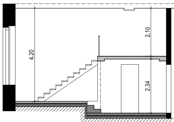
Prinzip-Querschnitt
