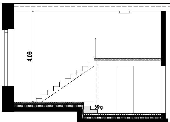
Prinzip-Querschnitt
