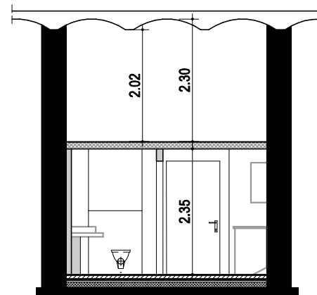
Prinzip-Längsschnitt
