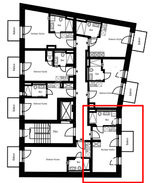
BAUTEIL B
