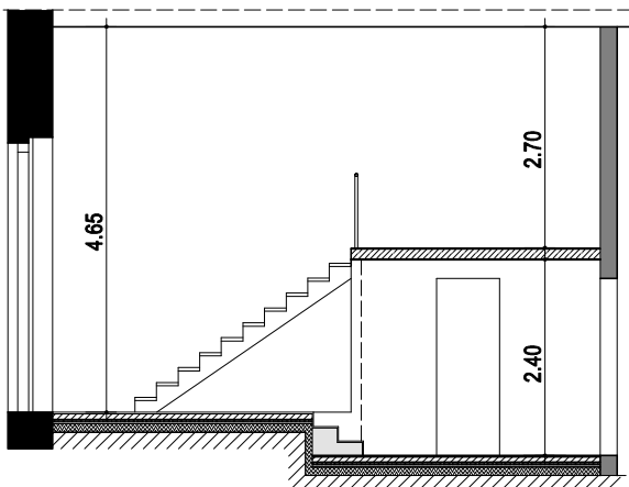
Prinzip-Querschnitt
