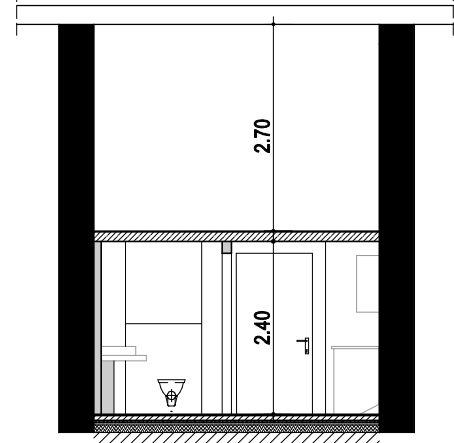
Prinzip-Längsschnitt
