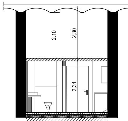
Prinzip-Längsschnitt
