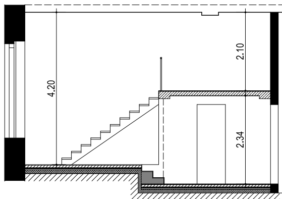
Prinzip-Querschnitt
